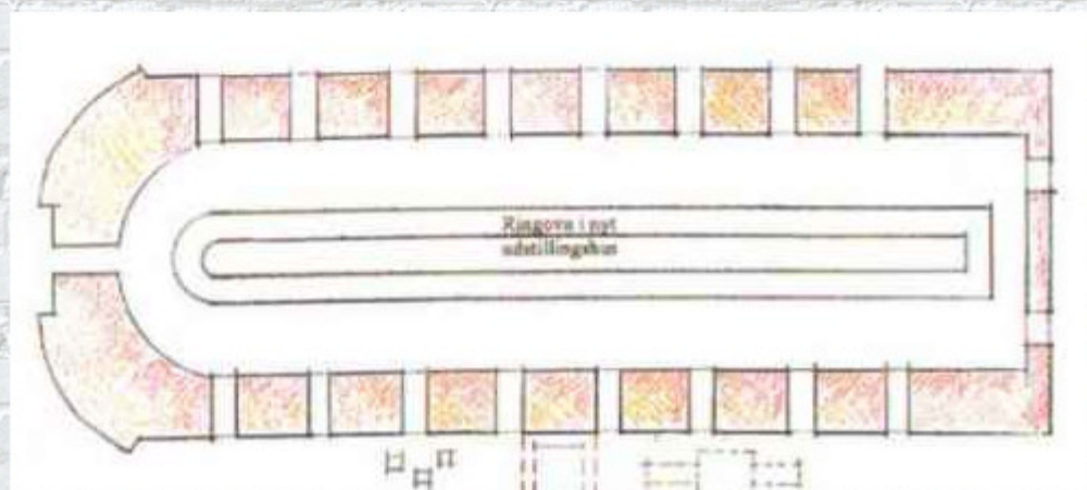
Tværsnit af Langhøjs Teglværks Ringovn.
